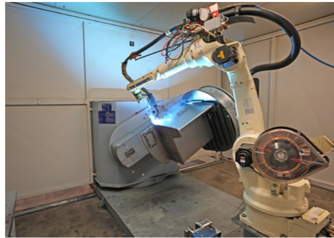
Die stahlbauliche Fertigung der Katzrahmen erfolgt mit Hilfe eines Schweißroboters. Dadurch sind kurze Durchlaufzeiten und gleichbleibende Schweißergebnisse gewährleistet.
